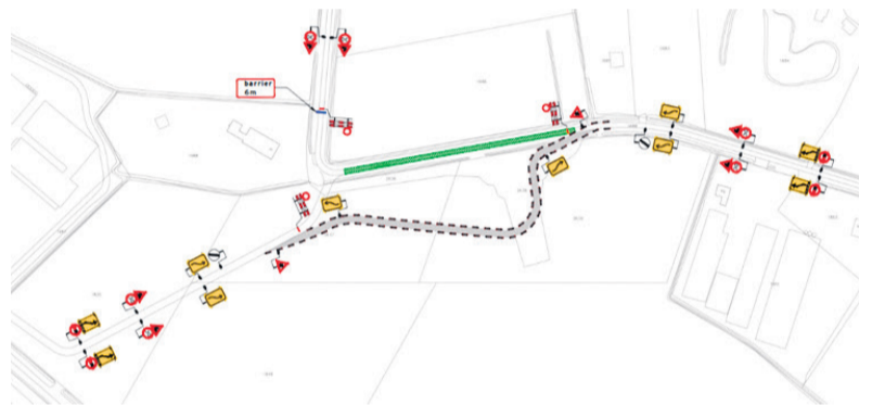
Verkeersmaatregelen rotonde Laverdonk
