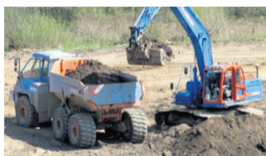
Laden dumper voor herschikking vrijkomende grond binnen het werk
